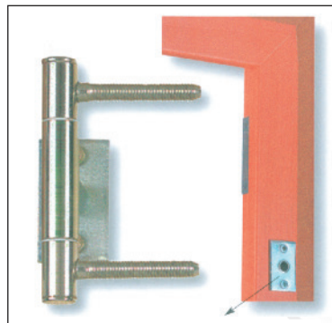
Montageplatte auf der Blendrahmenrückseite
